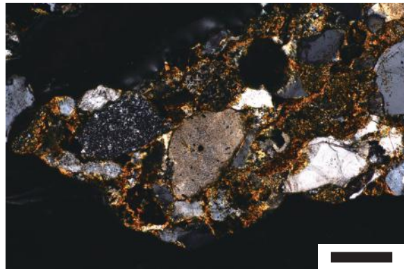
No.2、砂岩、直交ポーラ、スケールは 0.2mm
