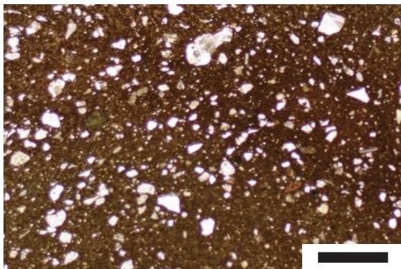
No.3 下方ポーラだけ、スケールは 2mm
