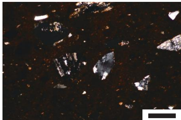
No.5、中央左は安山岩、中央右は多結晶石英、直交ポーラ、スケールは 0.2mm
