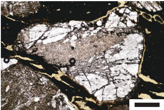
No. 1、中央はカタクレーサイト、下方ポーラだけ、スケールは 0.5mm
