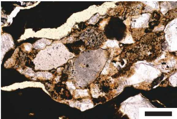
No.2、砂岩、下方ポーラだけ、スケールは 0.2mm
