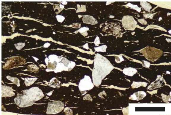
No.1 下方ポーラだけ、スケールは 2mm
