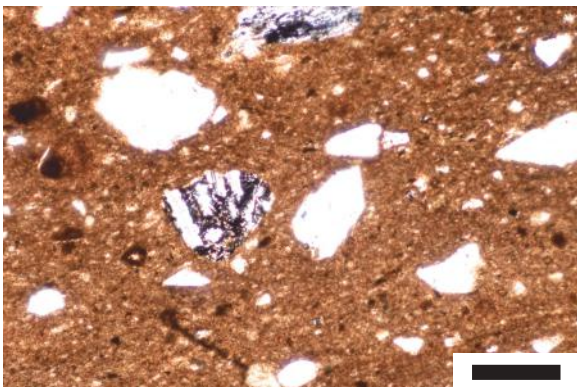
No.5、中央左は安山岩、中央右は多結晶石英、下方ポーラだけ、スケールは 0.2mm
