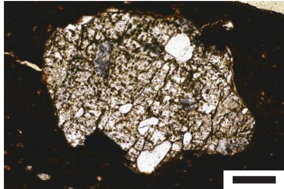
No.2、花崗岩類、下方ポーラだけ、スケールは 0.2mm
