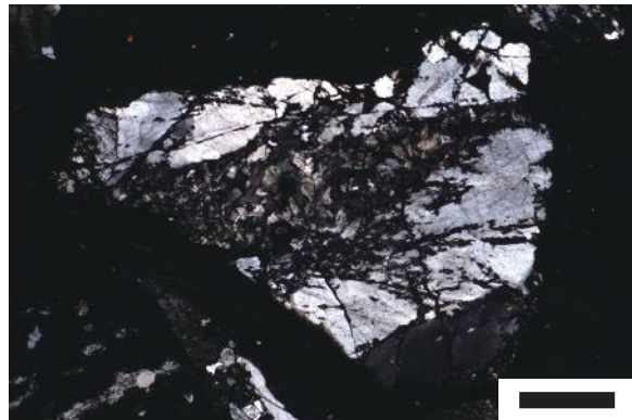
No.1、中央はカタクレーサイト、直交ポーラ、スケールは 0.5mm
